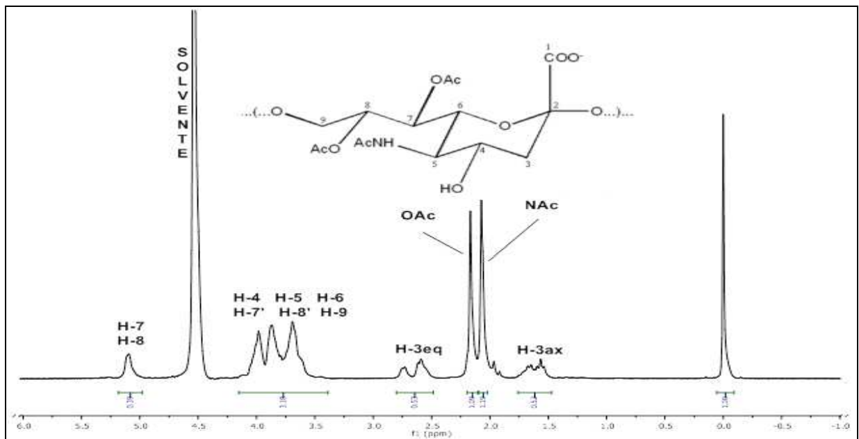
Figura 4.3 – Espectro de RMN de 1 H 400MHz, representativo para ambos os lotes analisados de PSC em D 2 O, com TSP- d 4 (0,0ppm). Lote: IMC0011.
