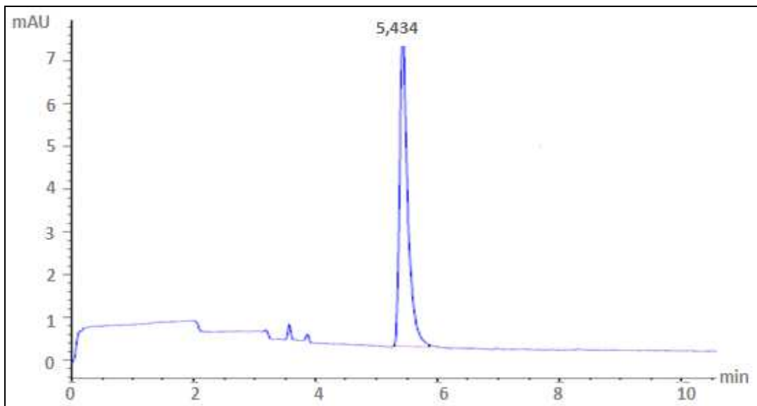
Figura 4.15- Eletroferograma referente à introdução da solução de galactose 500 \mu g/mL em tampão borato 20mM. Condições de análise descritas na Figura 4.13.
