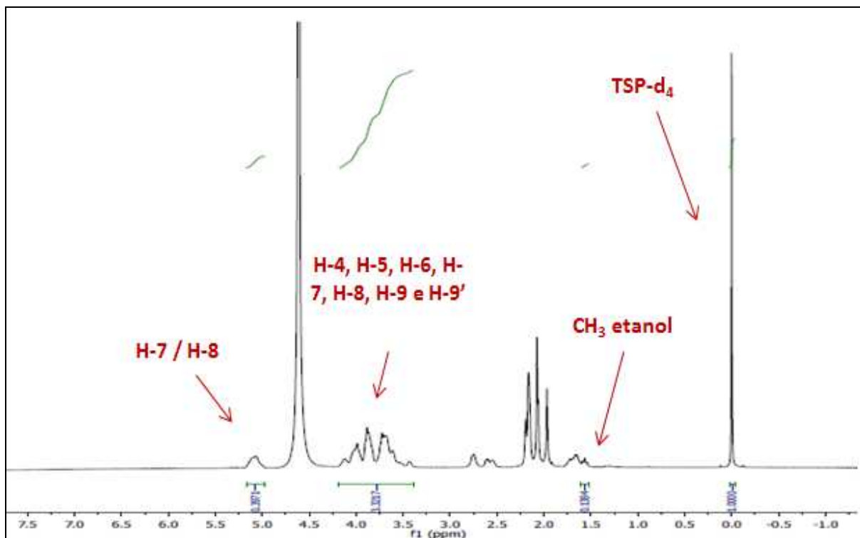
Figura 3.1 – Espectro de RMN de ^1H , 500MHz, do PSC em D2O com os sinais de interesse para quantificação integrados.
